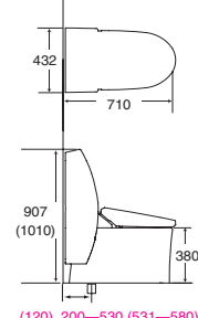
<Настенное устройство>
